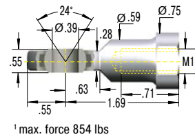
E10-VA Swivel Eye
