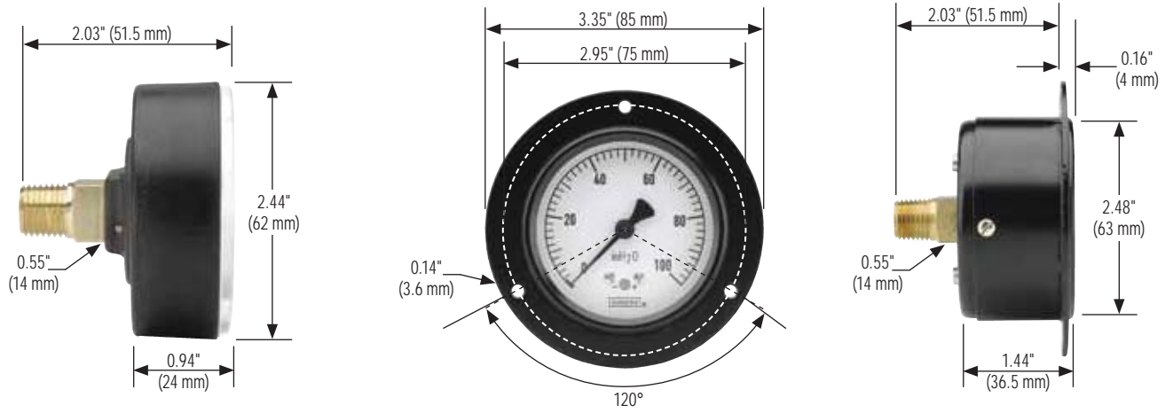
25-200 Rear Flange
